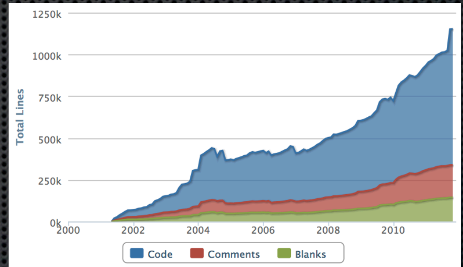
LLVM LOC
