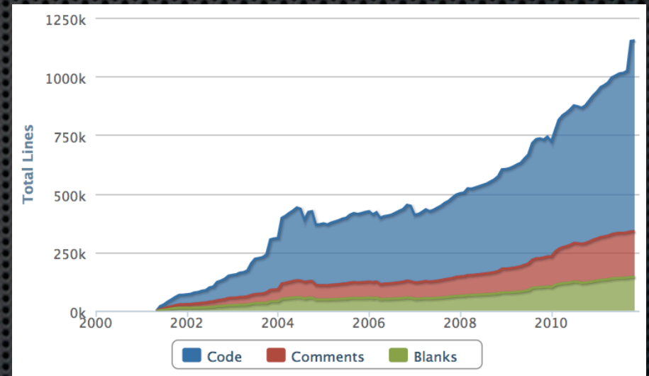
LLVM LOC
