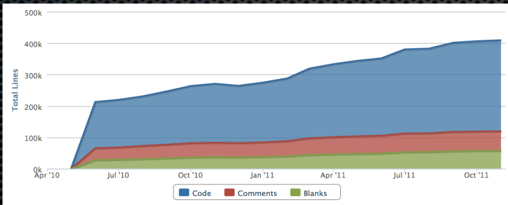
LLDB LOC
